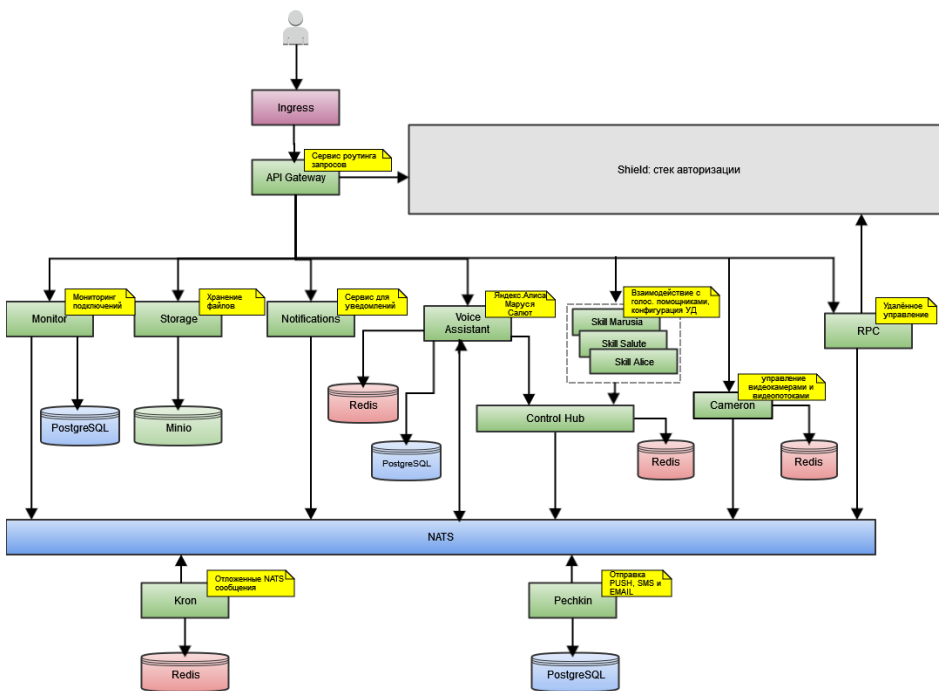
Рисунок 2 - схематичное изображение архитектуры SMHCloud
