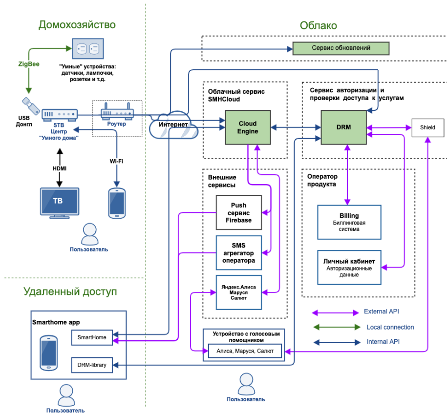
Рисунок 1 - схематичное представление взаимодействия компонентов "Умного дома" с использованием облачного сервиса SMHCloud
